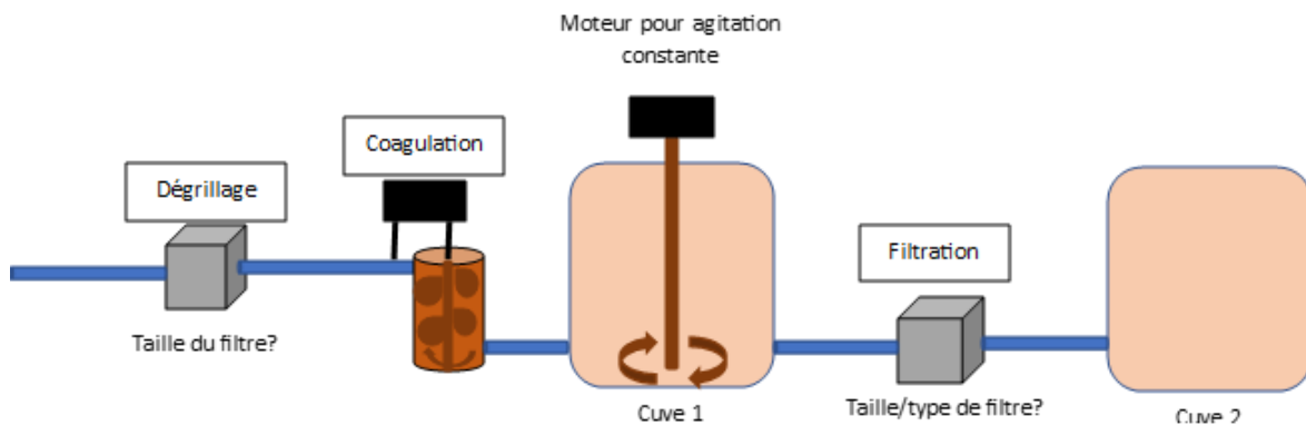
Schéma système
